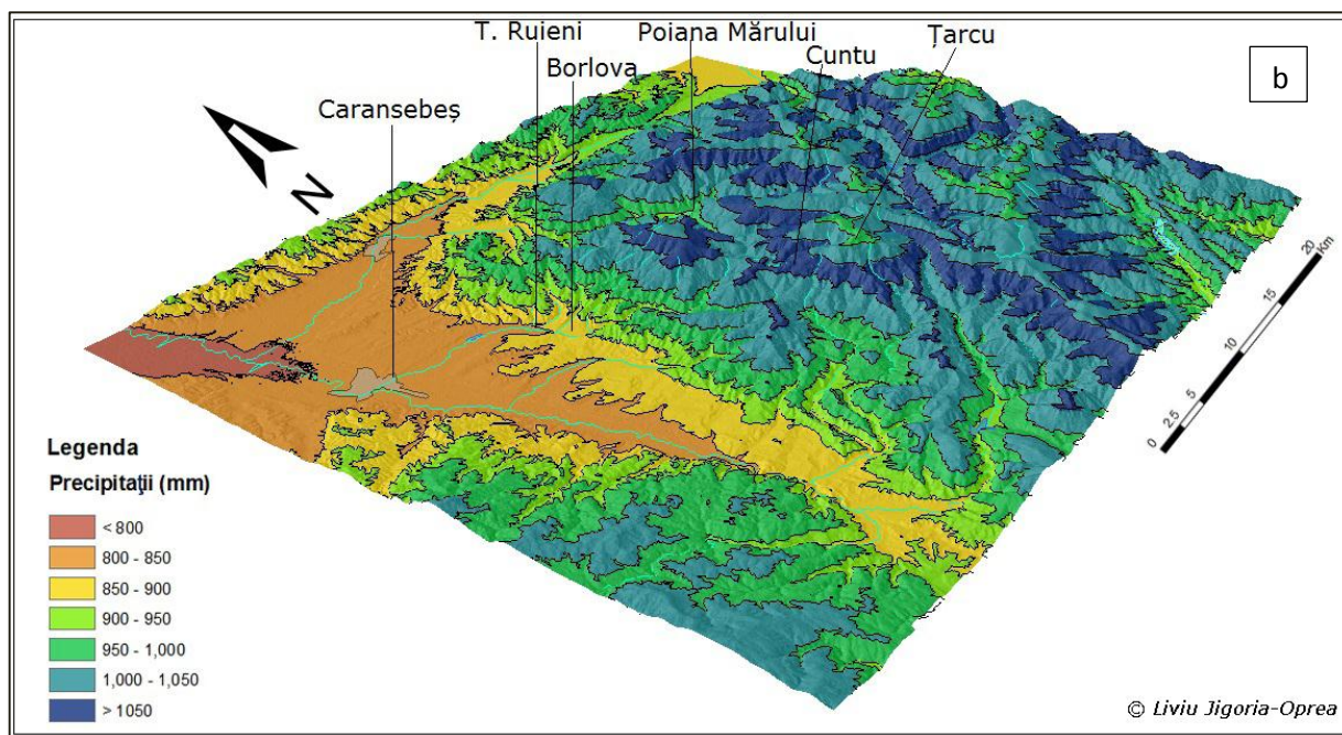
Fig. 2 – Temperatura medie anuală (a) și precipitațiile medii anuale (b) din Caransebeș și zona învecinată
